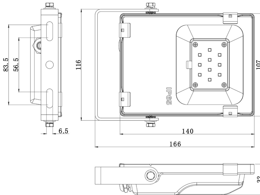
F105 Dimensions shown
